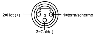
Connettore XLR a 3 poli (visto dal lato della saldatura)
