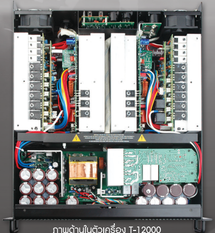
ภาพด้านในตัวเครื่อง T-12000
